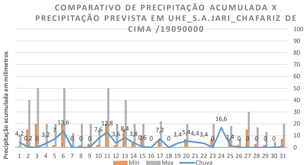
Gráfico 12: Precipitação acumulada (mm) estimada e registrada para o município de Laranjal do Jari (Estação ANA – Estação Meteorológica UHE Santo Antônio do Jari chafariz de cima) no mês de maio de 2016.
