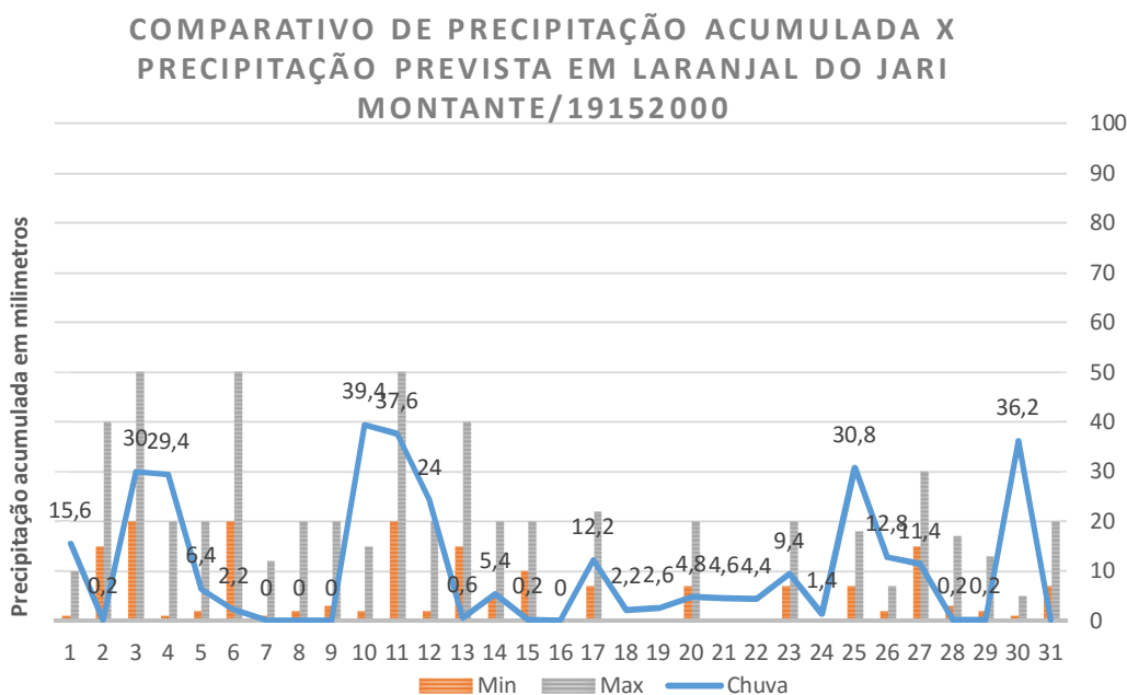
Gráfico 17: Precipitação acumulada (mm) estimada e registrada para o município de Porto Grande (Estação ANA – Estação Meteorológica UHE Santo Antônio do Jari - montante) no mês de maio de 2016.
