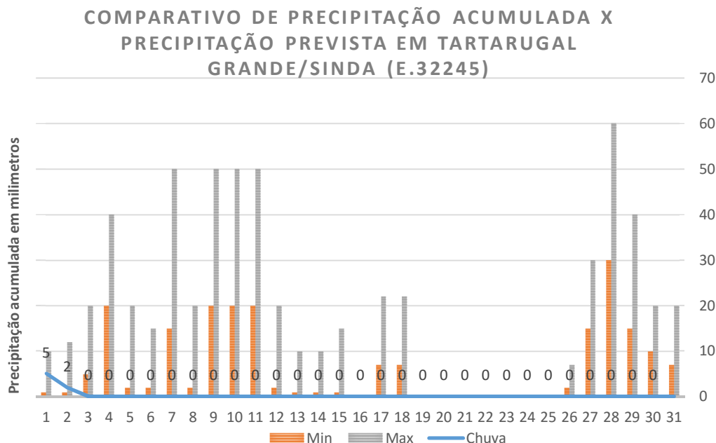
Gráfico 8: Precipitação acumulada (mm) estimada e registrada para o município de Tartarugalzinho (Estação ANA – Estação Meteorológica de Tartarugal Grande) no mês de maio de 2016.
