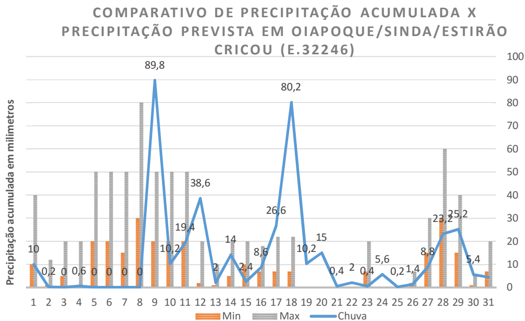
Gráfico 4: Precipitação acumulada (mm) estimada e registrada para o município de Oiapoque (Estação ANA – Estirão do Cricou) no mês de maio de 2016.
