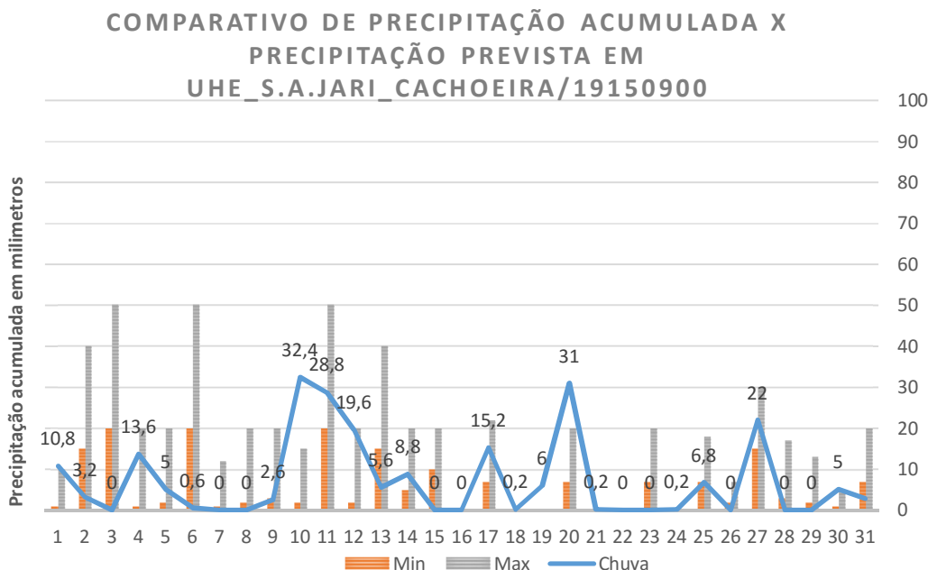
Gráfico 16: Precipitação acumulada (mm) estimada e registrada para o município de Porto Grande (Estação ANA – Estação Meteorológica UHE Santo Antônio do Jari - cachoeira) no mês de maio de 2016.
