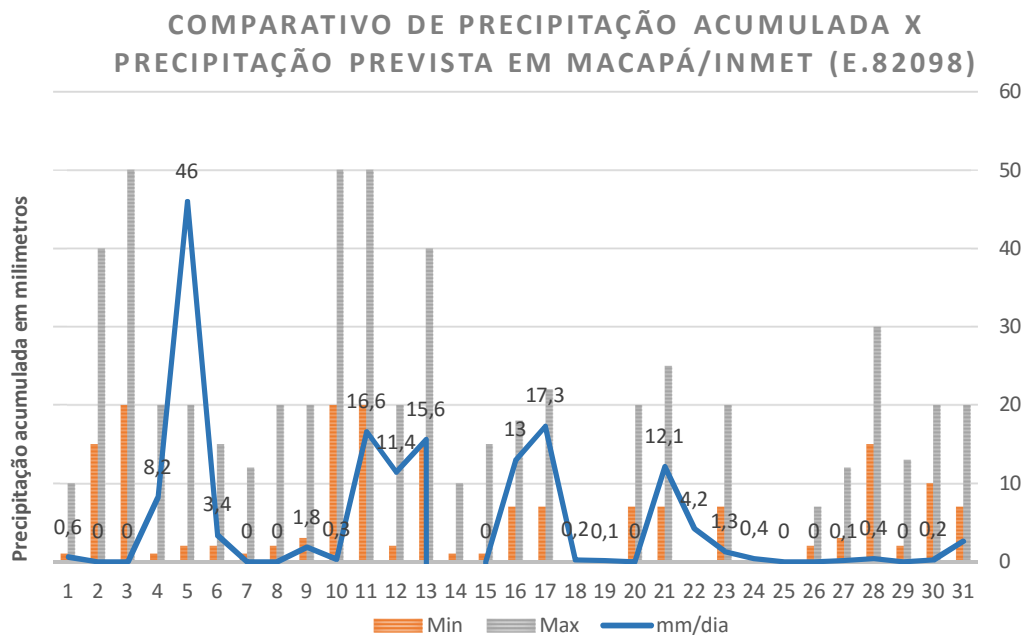
Gráfico 3: Precipitação acumulada (mm) estimada e registrada para o município de Macapá (Estação INMET - Fazendinha) no mês de maio de 2016.
