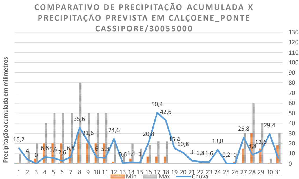
Gráfico 6: Precipitação acumulada (mm) estimada e registrada para o município de Calçoene (Estação ANA – Ponte do Cassiporé) no mês de maio de 2016.
