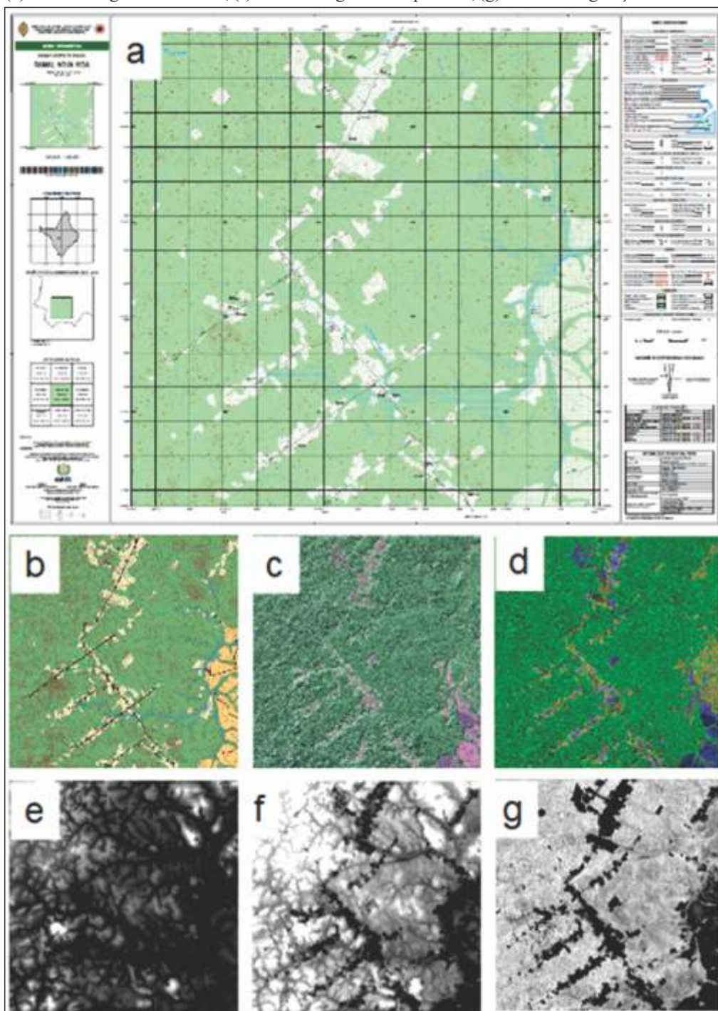
Figura 5 – Exemplos de produtos da BCDC-AP: (a) Carta topográfica folha MI 0160-3-SE-Ramal Nova Vida, escala 1:25.000; (b) produtos vetoriais em formato shapefile; (c) composição colorida das bandas X e P (produto BRADAR); (d) composição colorida das bandas X e P (produto EB); (e) Modelo Digital de Terreno, (f) Modelo Digital de Superfície, (g) altura da vegetação.
